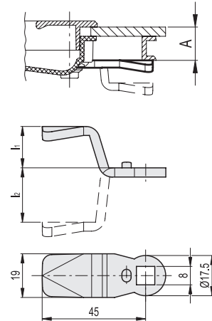
Montaggio su maniglia GN 115.10
