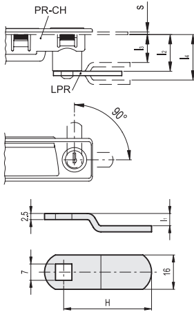
Montaggio su maniglia PR-CH
